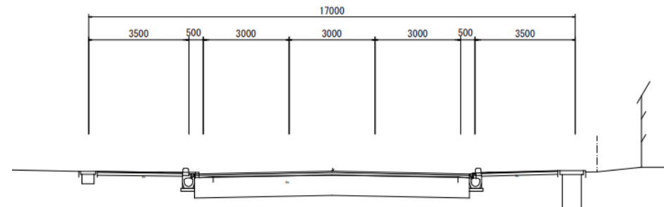
標準横断図 (南中里側道路部)
