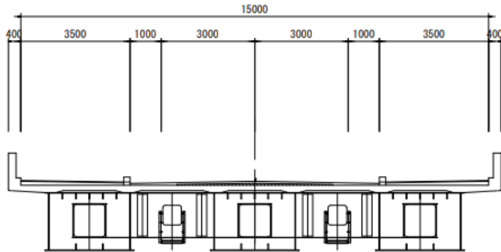
標準横断図 (橋梁部)
