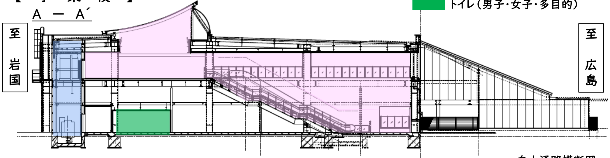
自由通路横断図
