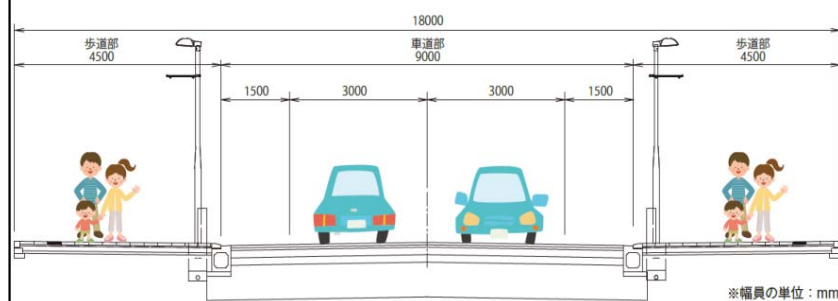
標準横断面
