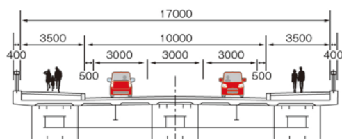
橋梁断面図
