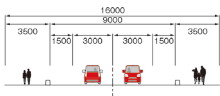
道路断面図
