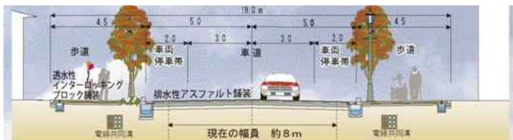
横断面図
